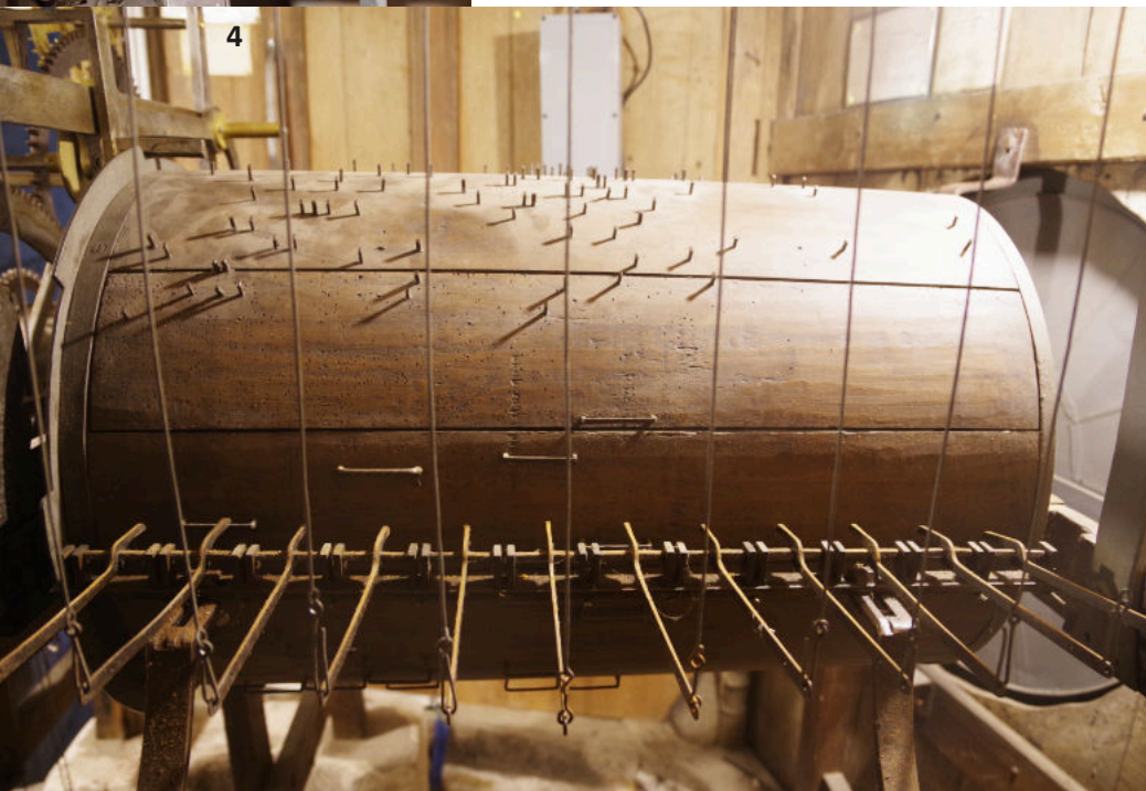
4 - Le cylindre des mélodies.
